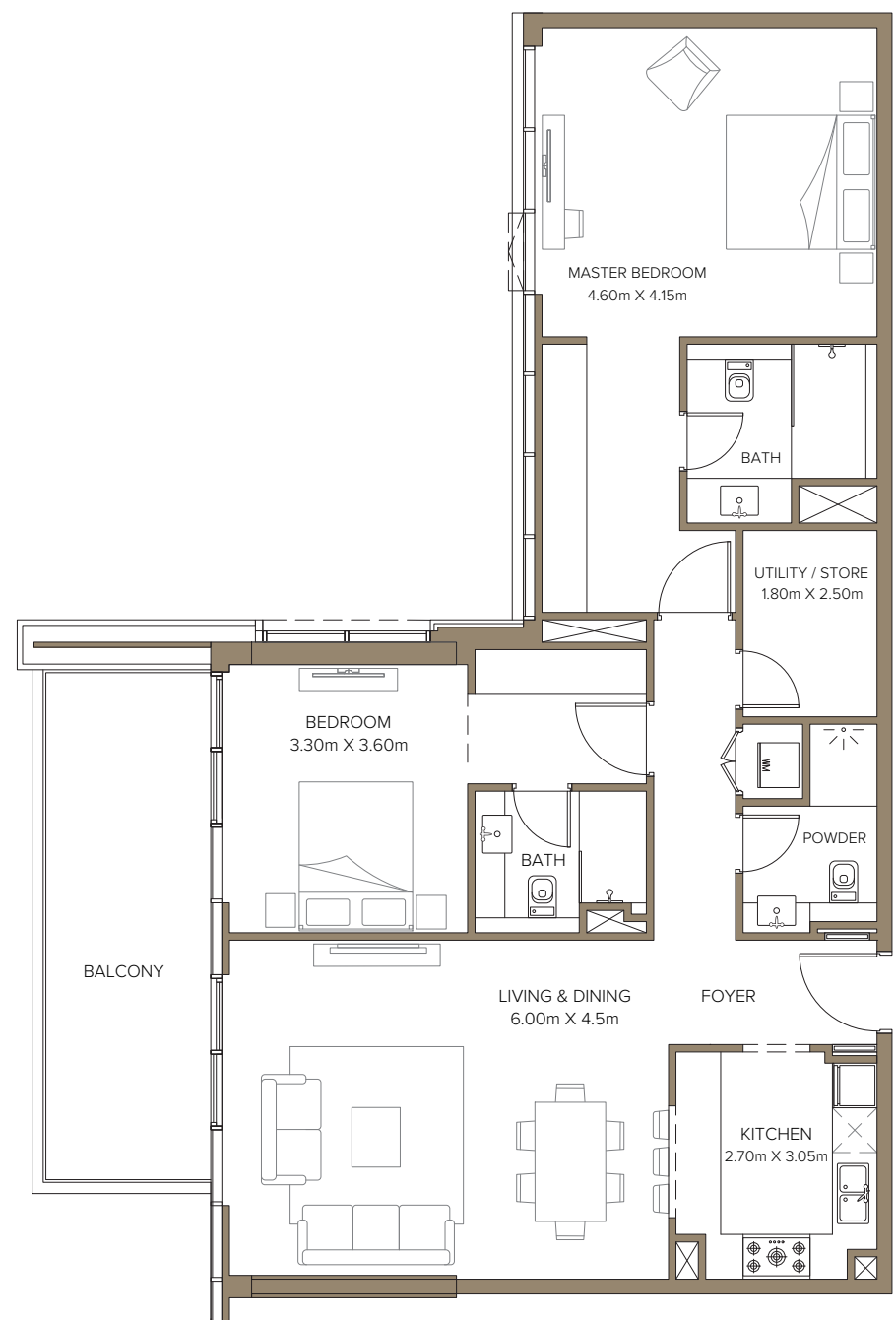
2B-E SCALE 1:100
